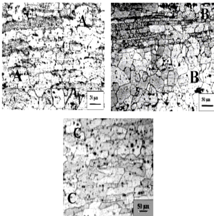
Figure 1: Microstructure des échantillons de l'alliage Al-6,2%Zn-2,5%Mg-1,7% Cu, A : Etat brut B : Etat Homogénéisé et C : Etat Homogénéisé et Déformé
