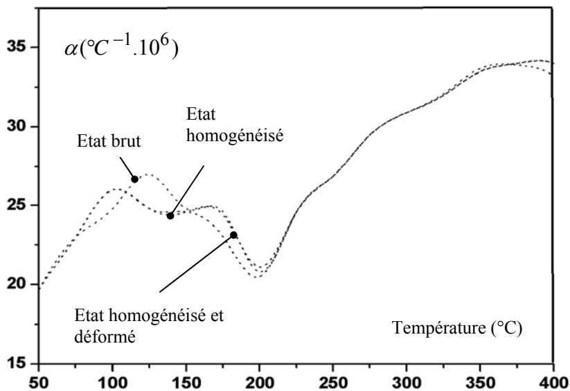
Figure 4 : Variation de \alpha en fonction de la température de l'alliage Al-6,2%Zn-2,5%Mg-1,7%Cu pour les trois états structuraux
