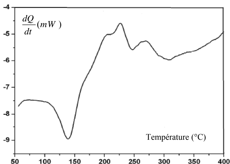
Figure 3 : Variation de la DCS en fonction de la température de l’alliage Al-6,2%Zn-2,5%Mg-1,7% Cu à l’état brut
