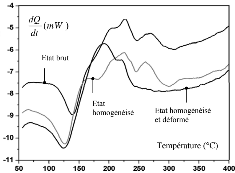
Figure 5 : Variation de la DCS en fonction de la température de l'alliage Al-6,2%Zn-2,5%Mg-1,7%Cu, pour les trois états structuraux
