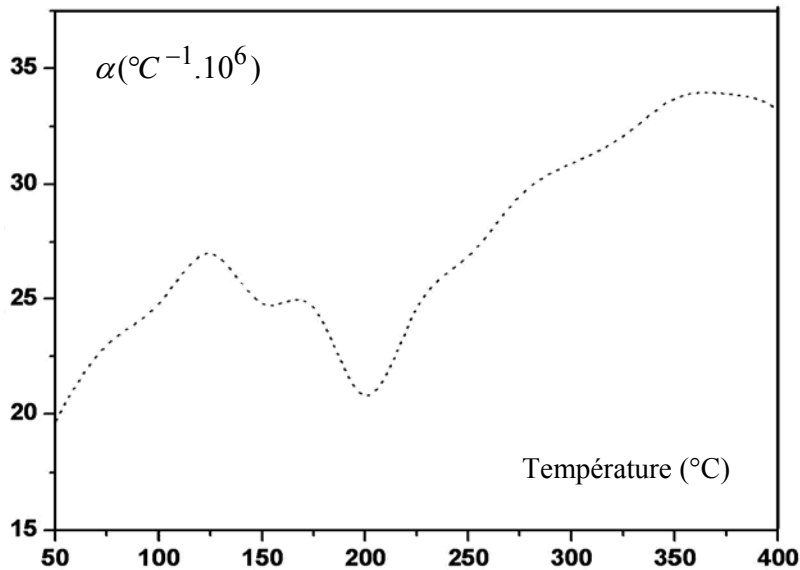
Figure 2 : Variation de \alpha en fonction de la température de l'alliage Al-6,2% Zn-2,5% Mg-1,7% Cu à l'état brut
