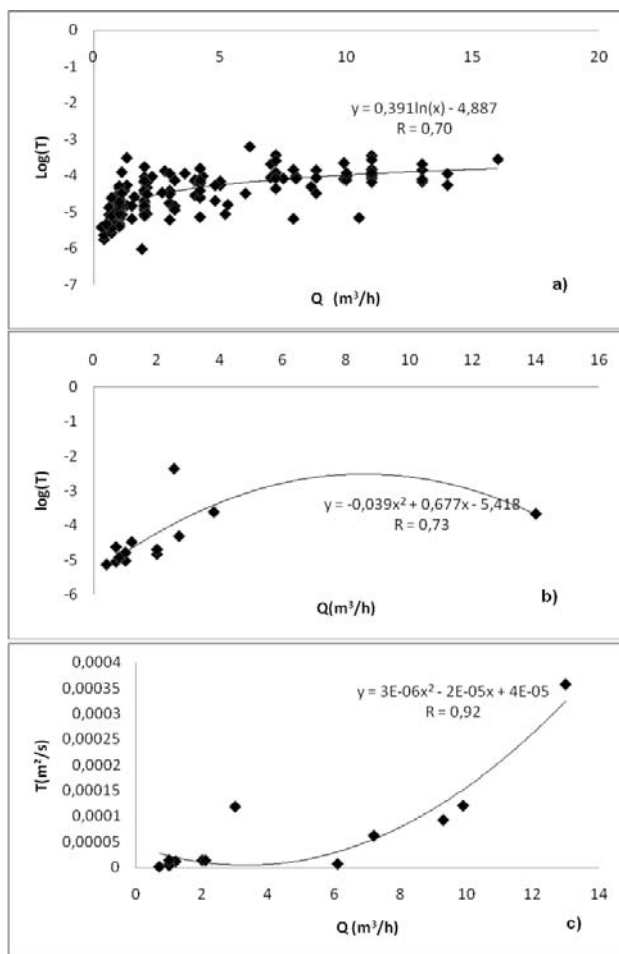
Figure 6: Transmissivité en fonction du débit de forage dans les formations métamorphiques (a), les granites (b) et les grès (c).
