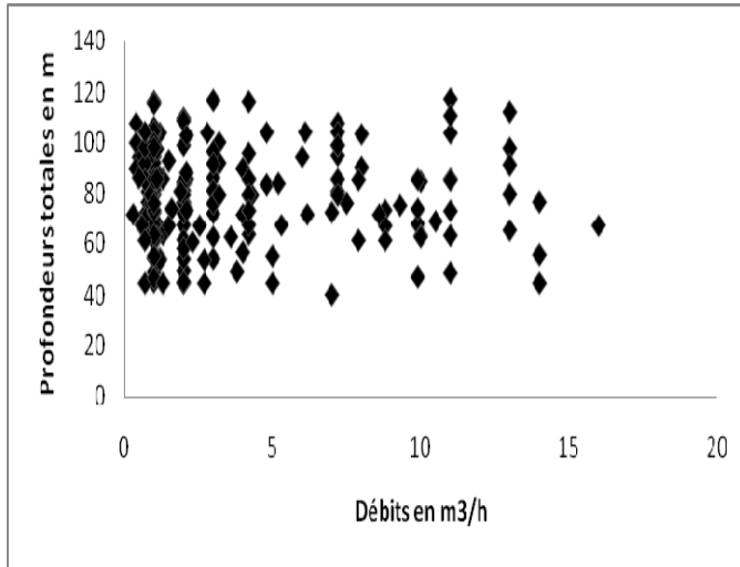
Figure 3: Evolution des débits en fonction des profondeurs totales des forages
