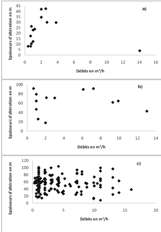
Figure 5: Evolution des débits en fonction des épaisseurs d'altérites dans les granites (a), les grès (b) et les formations métamorphiques (c)
