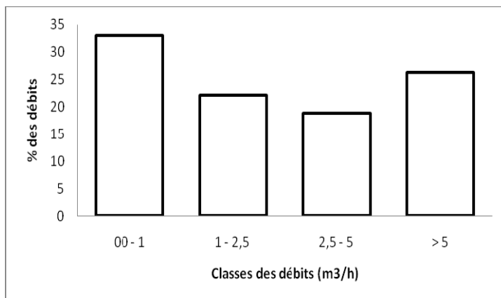
Figure 2: Distribution des débits en fonction des classes
