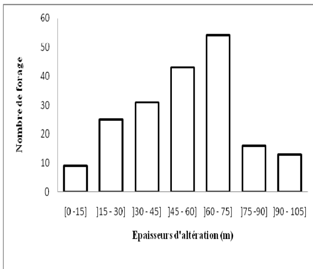
Figure 4: Fréquence de la distribution de la puissance des altérations dans la région N'zi-Comoé
