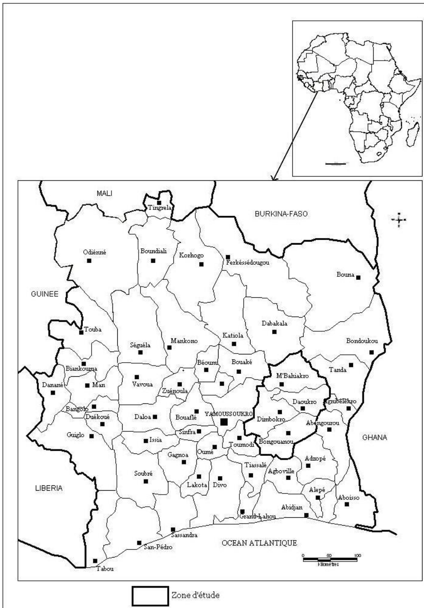
Figure 1 : Localisation de la région du N'zi-Comoé (Centre-Est de la Côte d'Ivoire)
